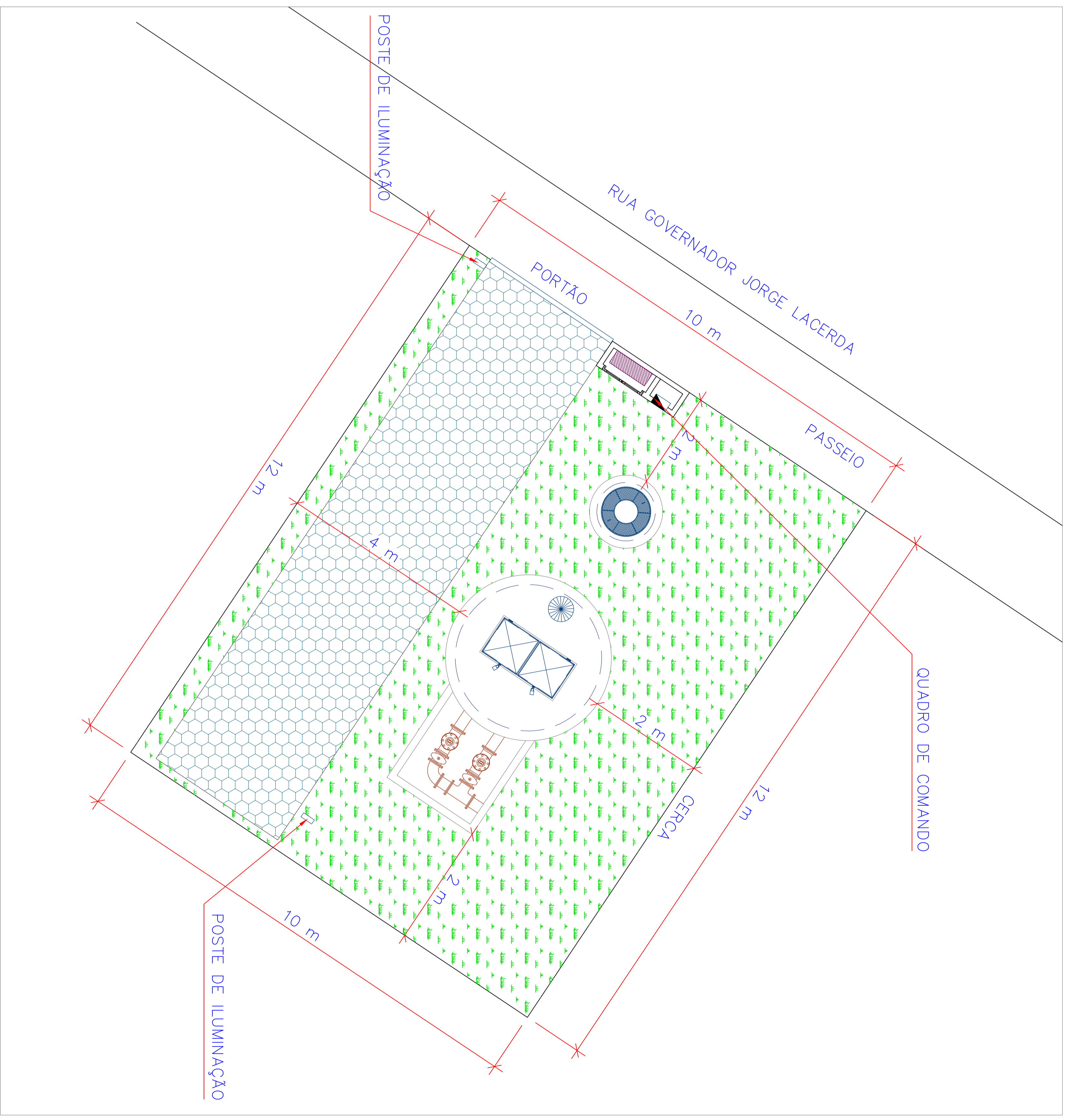
2 PLANTA DE LOCALIZAÇÃO E URBANIZAÇÃO ESCALA 1:500
