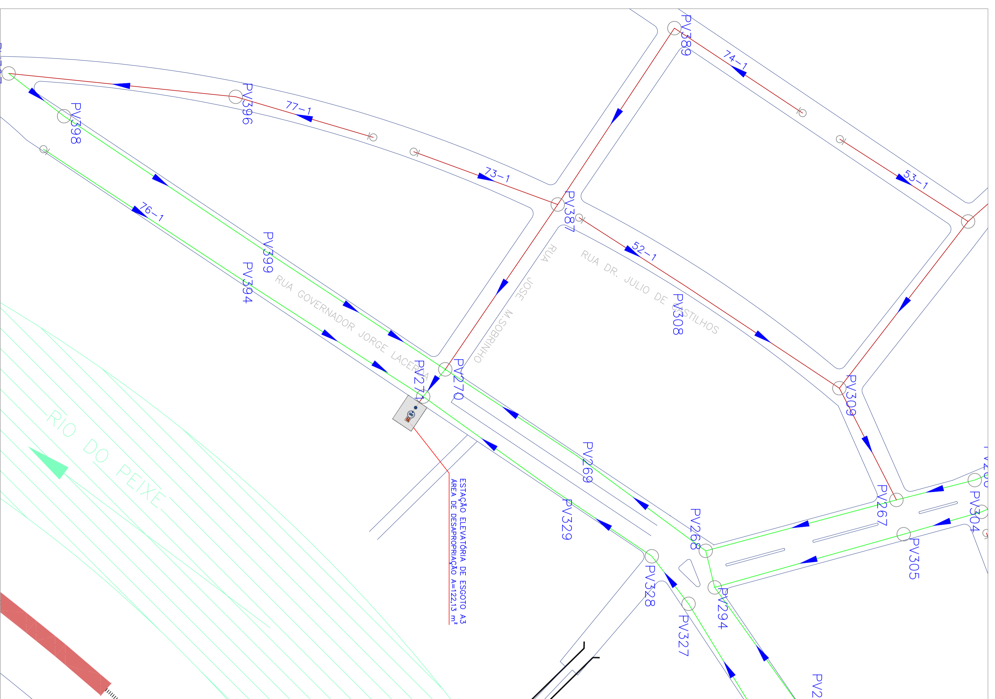
1 PLANTA DE SITUAÇÃO ESCALA 1:1000
