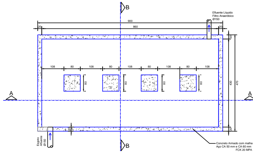
PLANTA BAIXA
