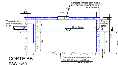
SISTEMA DE FOSSA SÉPTICA DISTRITO DE SANTA LÚCIA - OURO - SC
