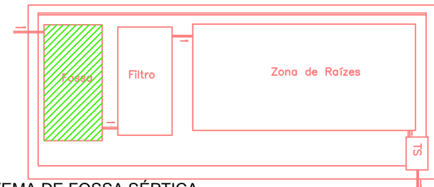
SISTEMA DE FOSSA SÉPTICA DISTRITO DE SANTA LÚCIA - OURO - SC
