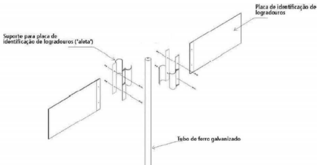
Figura 2 - Detalhe Fixação Placas
