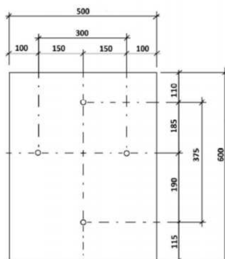
PLACA 0,50 x 0,60 m
