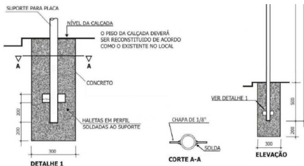
Figura 4 - Detalhe do Dispositivo Anti-Giro e da Fundação
