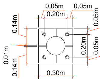
DETALHE DO CHUMBAMENTO ESCALA 1/20
