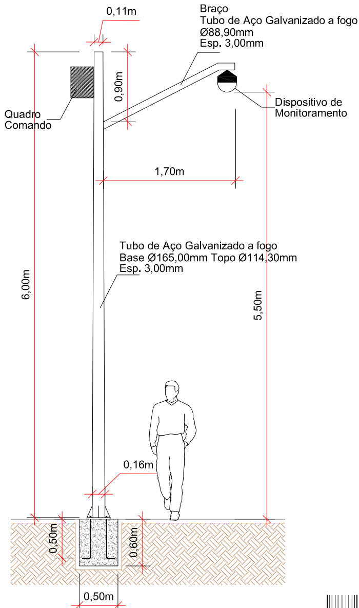
DETALHE DO POSTE ESCALA 1/50
